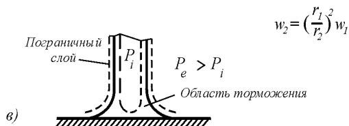
Рис. 4.8. Вращение тела: вокруг цилиндра (а); вокруг центра при изменении радиуса вращения (б); структура нижней части смерча, в которой газ движется с изменением радиуса вращения (в)
