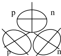
Рис. 1.23. Структура ядра {}_6\text{C}^{12}
