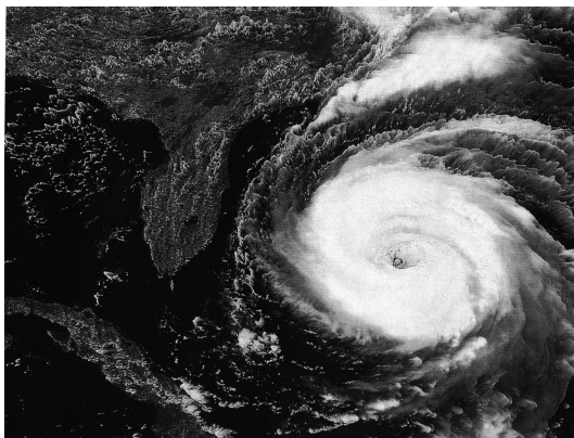
Рис. 4.6. Образование циклона в районе Флориды (снимок из космоса)
