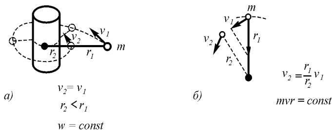
Рис. 4.7. Движение тела по траектории с переменным радиусом: без подвода энергии (а); с подводом энергии (б); к расчету центростремительного ускорения (в)
