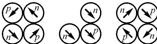
Рис. 1.21. Структура ядра {}_5B^{11}
