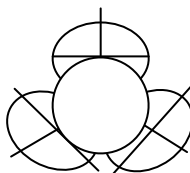
Рис. 1.24. Структура ядра {}_8\text{O}^{16}
